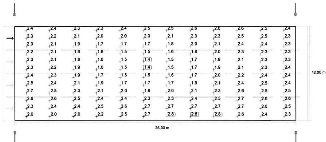
Observator 4: Densitatea luminii la instalația nouă [cd/m²] (Raster valoric)
