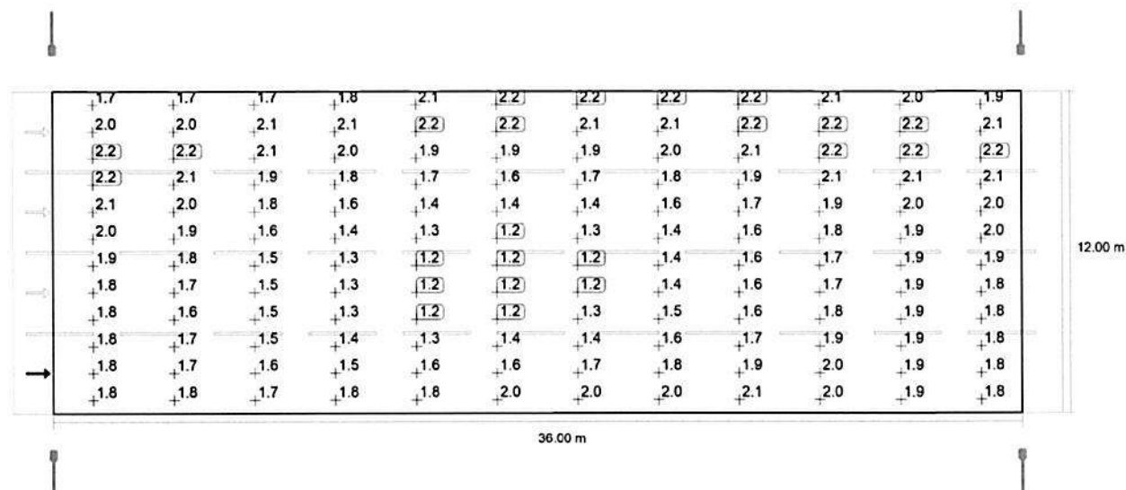
Observator 1: Valoarea de întreținere, densitatea luminii cu carosabil uscat [cd/m²] (Raster valoric)
