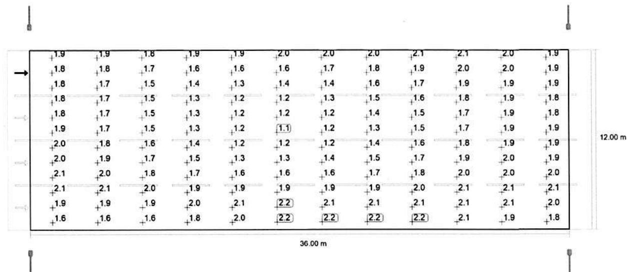
Observator 4: Valoarea de întreținere, densitatea luminii cu carosabil uscat [ \text{cd/m}^2 ] (Raster valoric)
