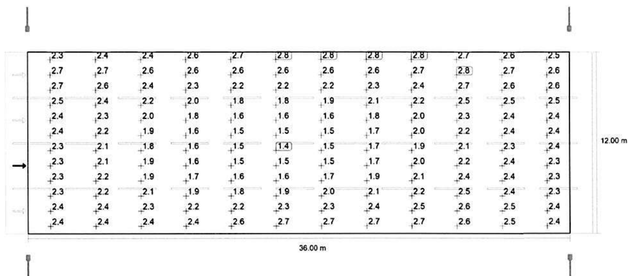
Observator 2: Densitatea luminii la instalația nouă [cd/m²] (Raster valoric)
