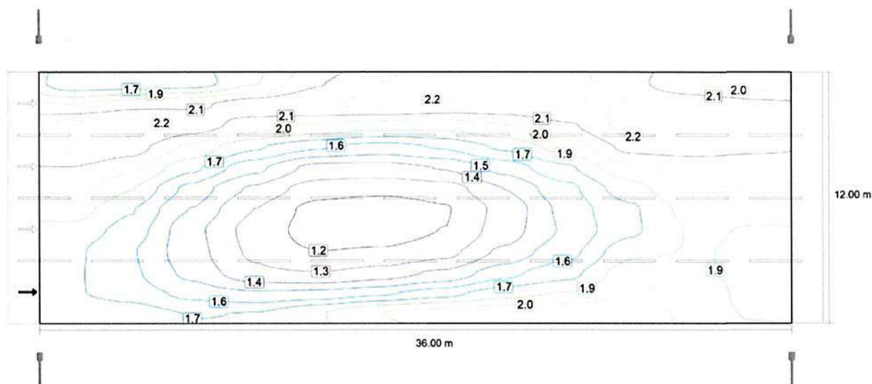
Observator 1: Valoarea de întreținere, densitatea luminii cu carosabil uscat [cd/m²] (Linii Isolux)
