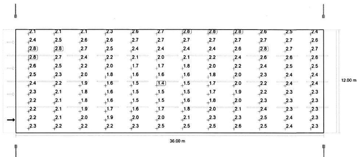
Observator 1: Densitatea luminii la instalația nouă [cd/m²] (Raster valoric)
